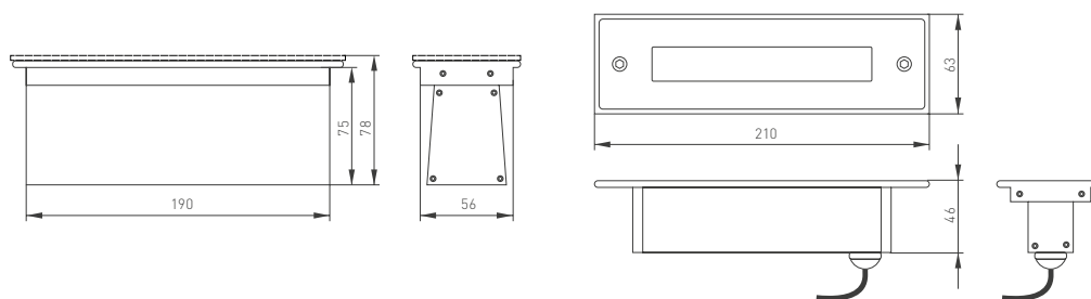
Рис. 1. Чертеж и габаритные размеры светильника
